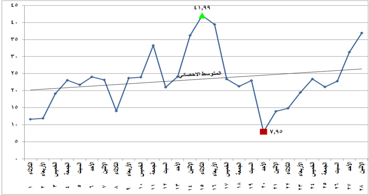
شكل (٢٥) الطاقة الكهربائية المنتجة من الرياح والشمس خلال شهر فبراير ٢٠٢٢
