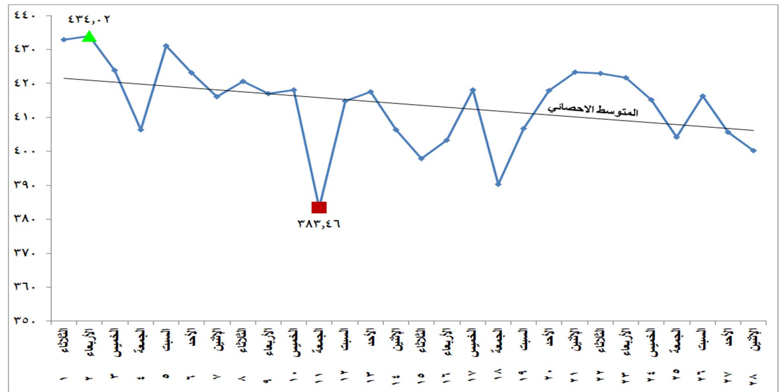
شكل (١٧) الطاقة الكهربائية المنتجة من الغاز الطبيعي خلال شهر فبراير ٢٠٢٢
