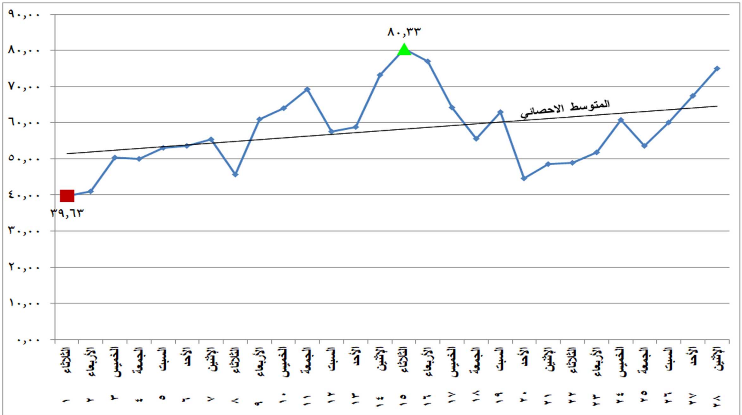
شكل (٢١) الطاقة الكهربائية المنتجة من المصادر غير الحرارية خلال شهر فبراير ٢٠٢٢
