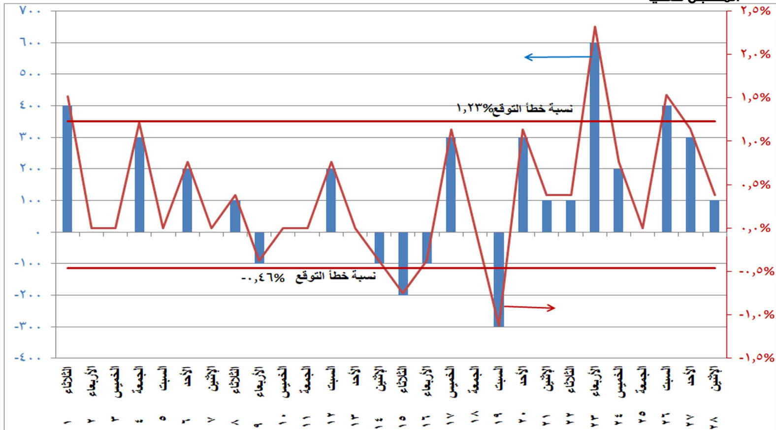
شكل (١٠) الفرق بين الحمل الأقصى المتوقع والمسجل فعليا ونسبة الفرق إلى الحمل المسجل فعليا خلال شهر فبراير ٢٠٢٢
