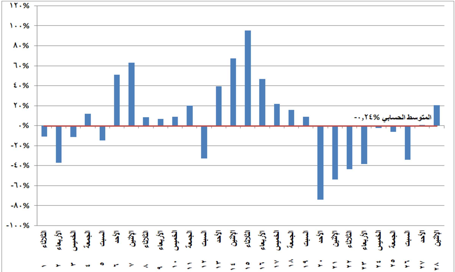
شكل (٢٦) نسب التغير في استخدام الرياح والشمس في إنتاج الطاقة الكهربائية خلال شهر فبراير ٢٠٢٢ مقارنة بالشهر المماثل من العام السابق
