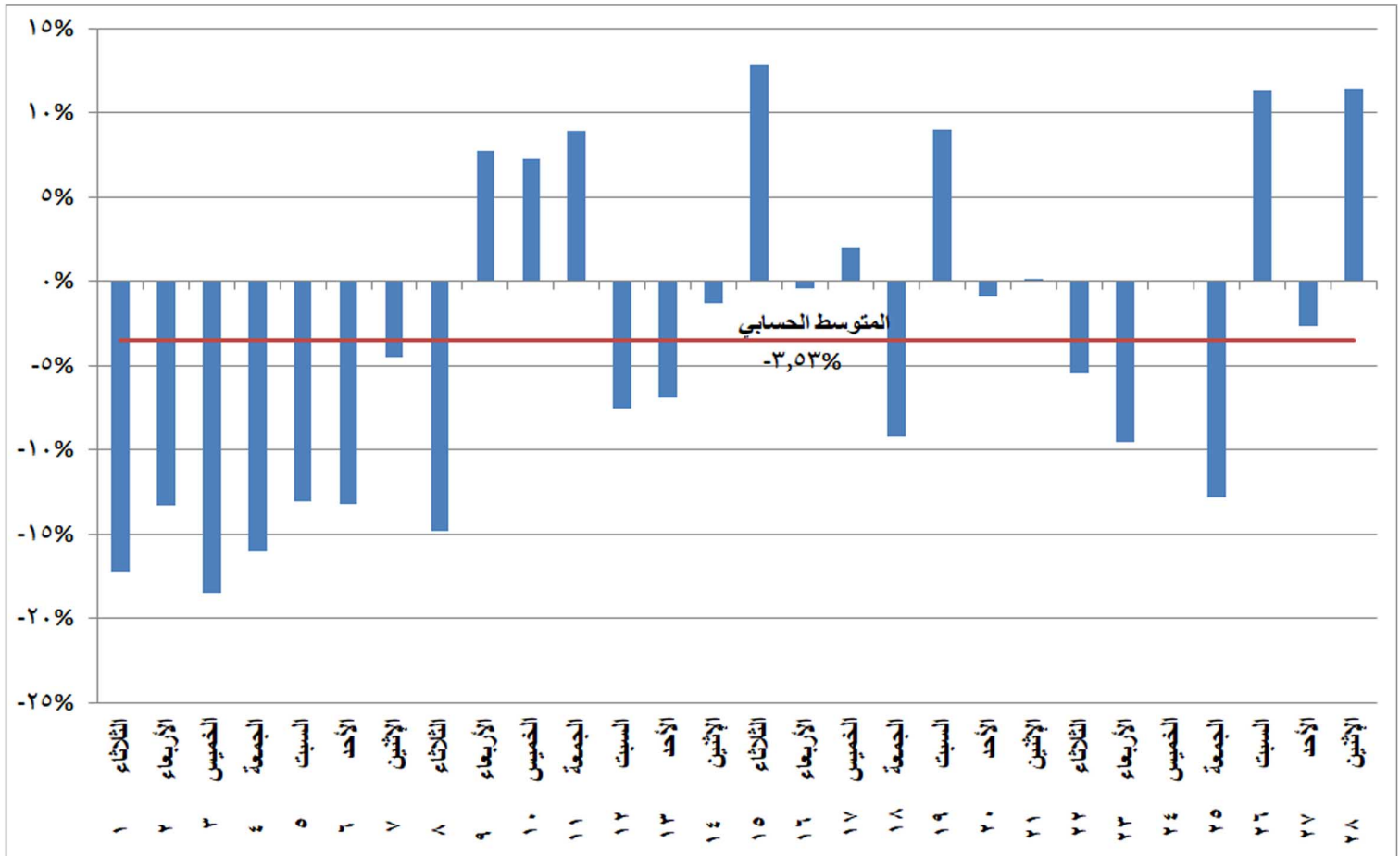
شكل (٢٤) نسب التغير في استخدام المصادر المائية في إنتاج الطاقة الكهربائية خلال شهر فبراير ٢٠٢٢ مقارنة بالشهر المماثل من العام السابق
