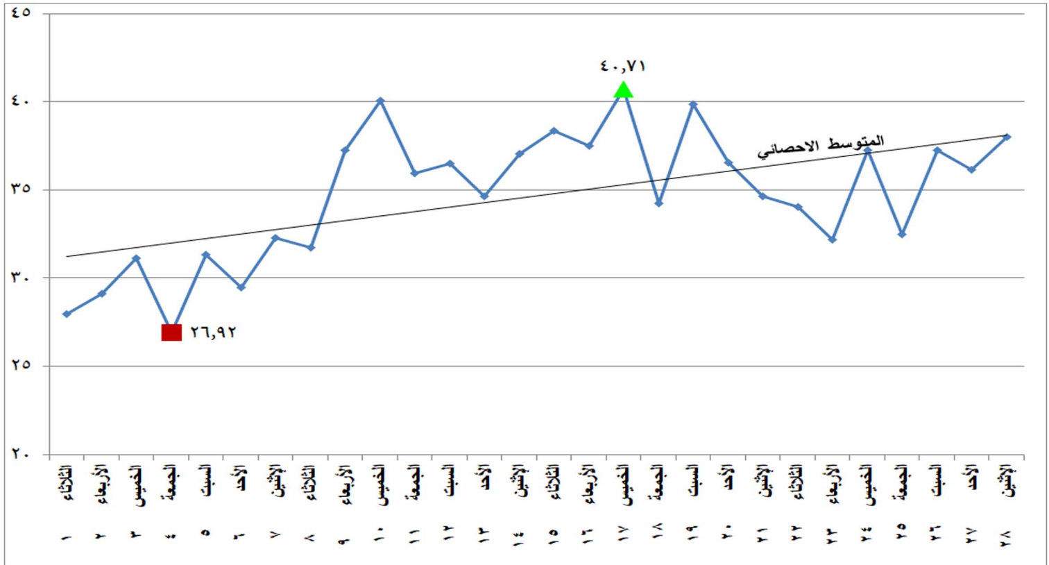
شكل (٢٣) الطاقة الكهربائية المنتجة من المصادر المائية خلال شهر فبراير ٢٠٢٢
