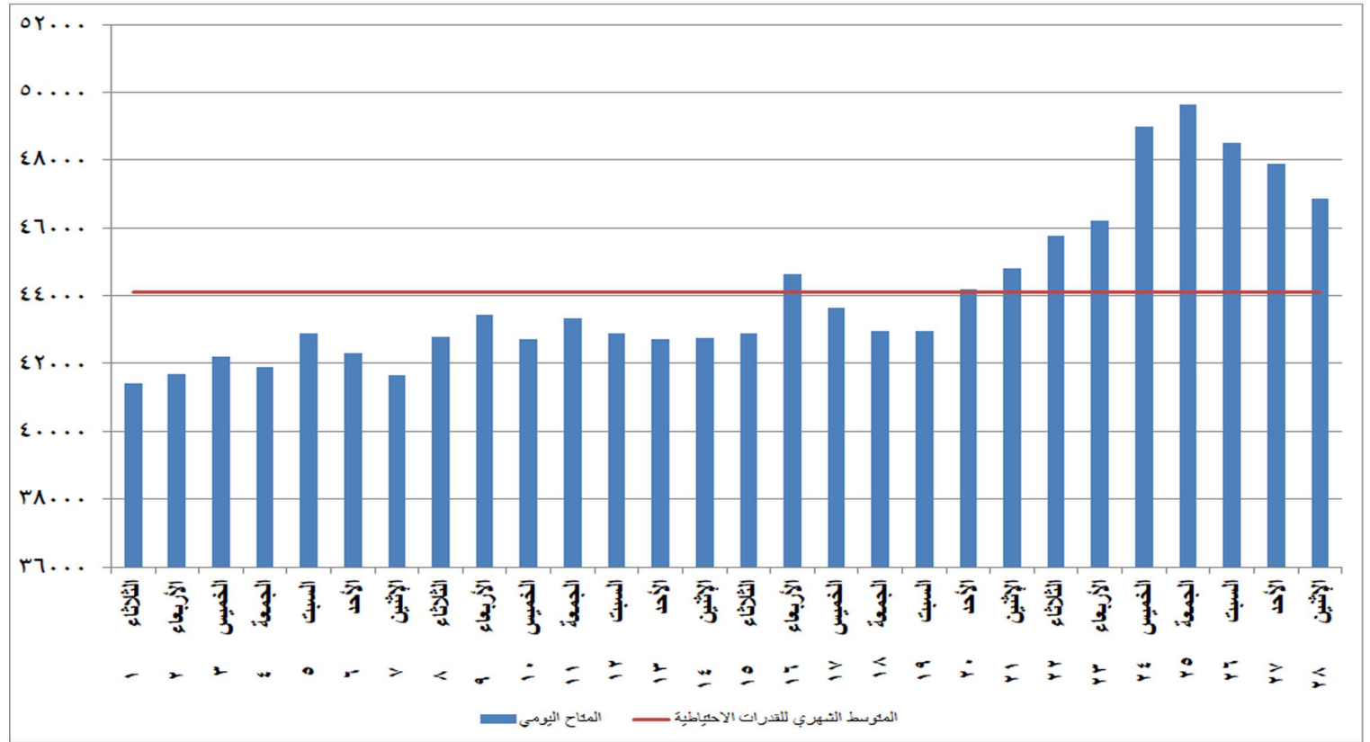
شكل (٢٧) القدرات المتاحة يوميا والمتوسط الشهري للقدرات الاحتياطية خلال شهر فبراير ٢٠٢٢
