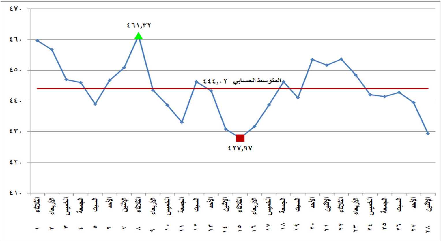
شكل (١٤) معامل انبعاثات غاز ثاني اكسيد الكربون المكافئ على مدى شهر فبراير ٢٠٢٢
