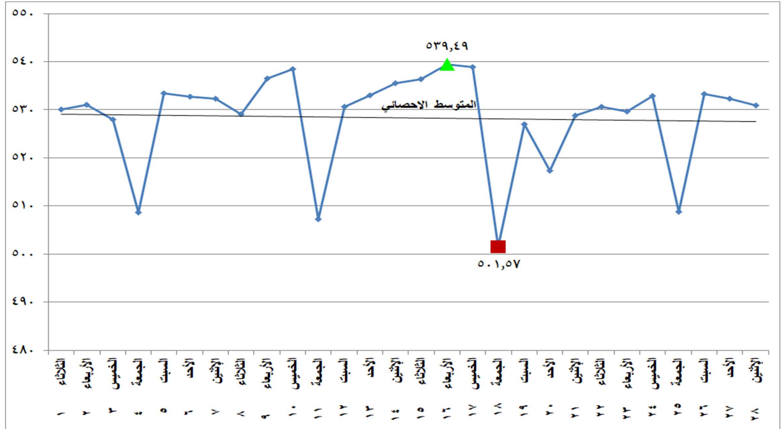
شكل (١٥) إجمالي الطاقة الكهربائية المنتجة من كل المصادر الأولية خلال شهر فبراير ٢٠٢٢
