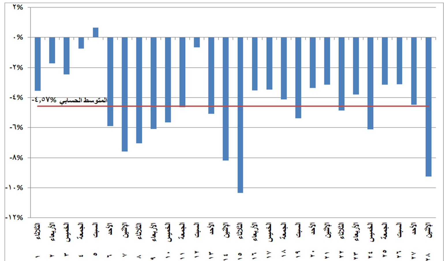
شكل (١٨) نسب التغير في استخدام الغاز الطبيعي في إنتاج الطاقة الكهربائية خلال شهر فبراير ٢٠٢٢ مقارنة بالشهر المماثل من العام السابق
