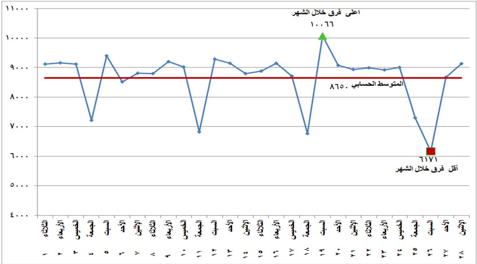
شكل (٣) الفرق بين أقصى وأدنى حمل خلال شهر فبراير ٢٠٢٢
