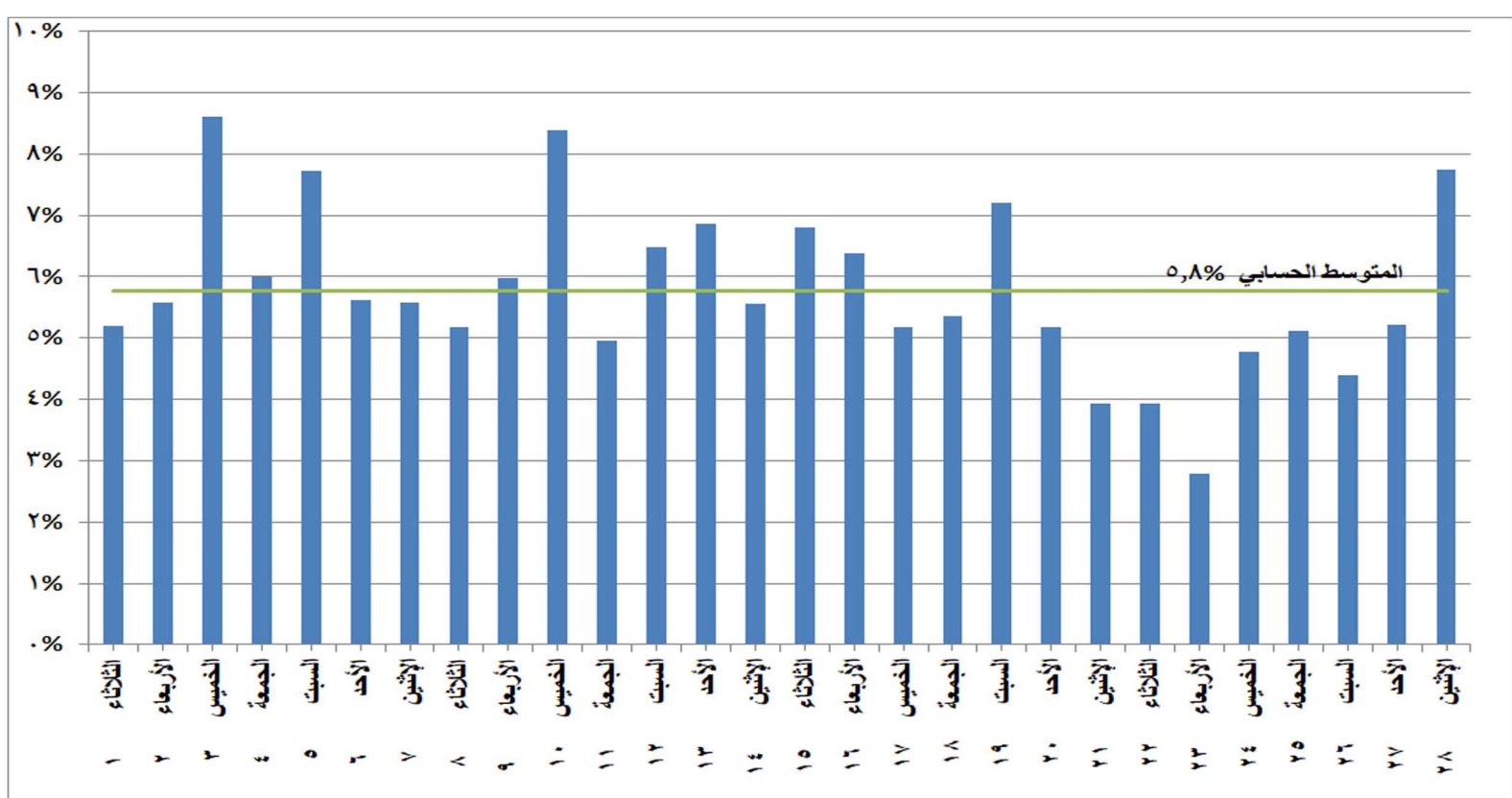
شكل (٩) النسب المئوية للتغير في الحمل الاقصى خلال شهر فبراير ٢٠٢٢ مقارنة باليوم المماثل من العام الماضي
