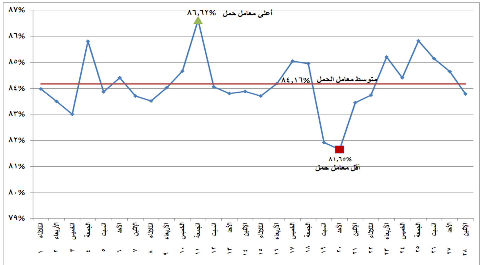
شكل (١٢) إجمالي معامل الحمل لوحدات الانتاج خلال شهر فبراير ٢٠٢٢
