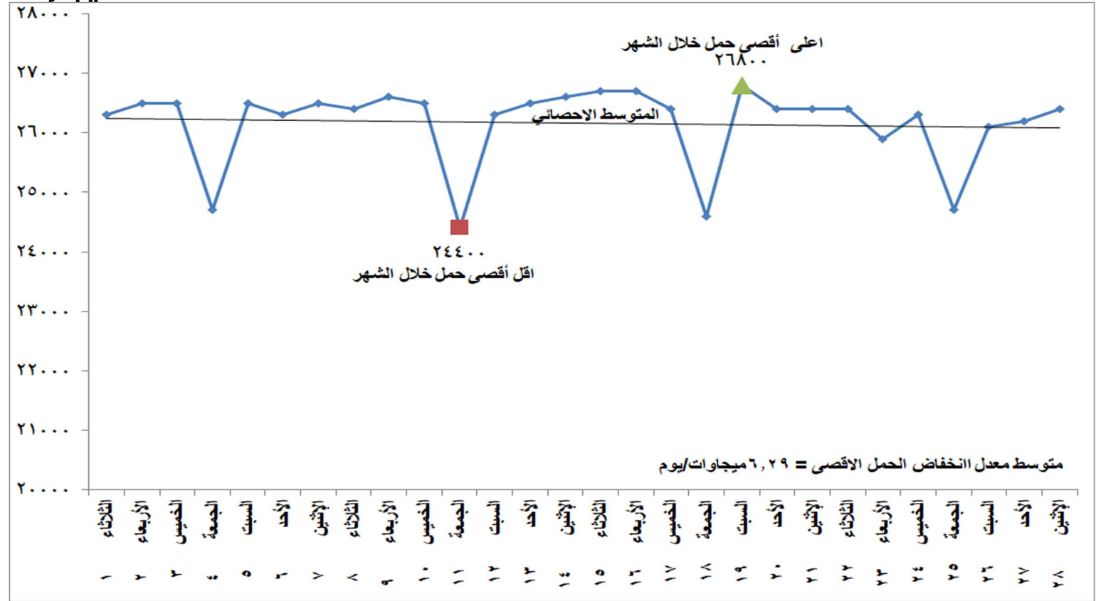
شكل (١) تطور الحمل الاقصى اليومي خلال شهر فبراير ٢٠٢٢
