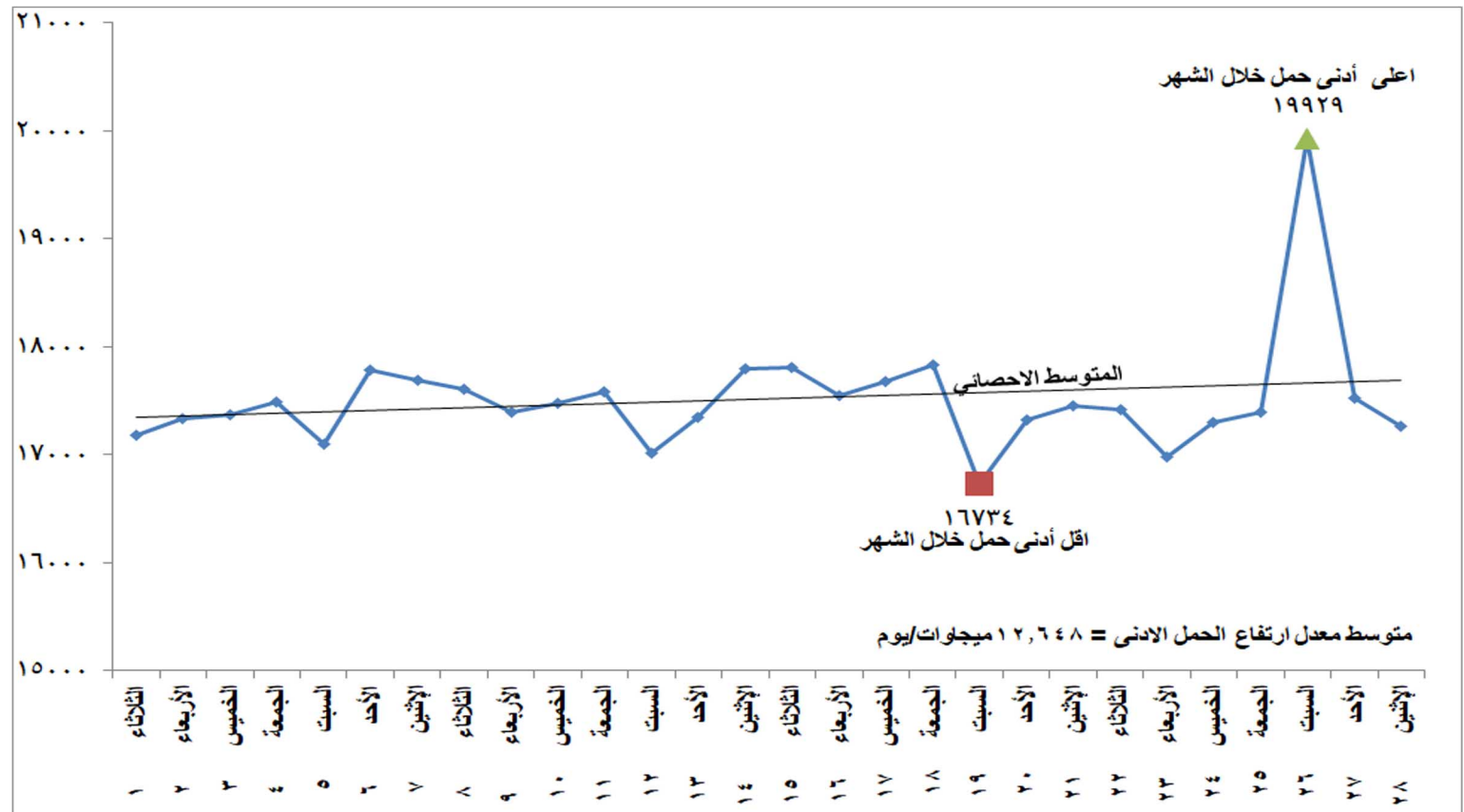
شكل (٢) تطور الحمل الادنى اليومي خلال شهر فبراير ٢٠٢٢
