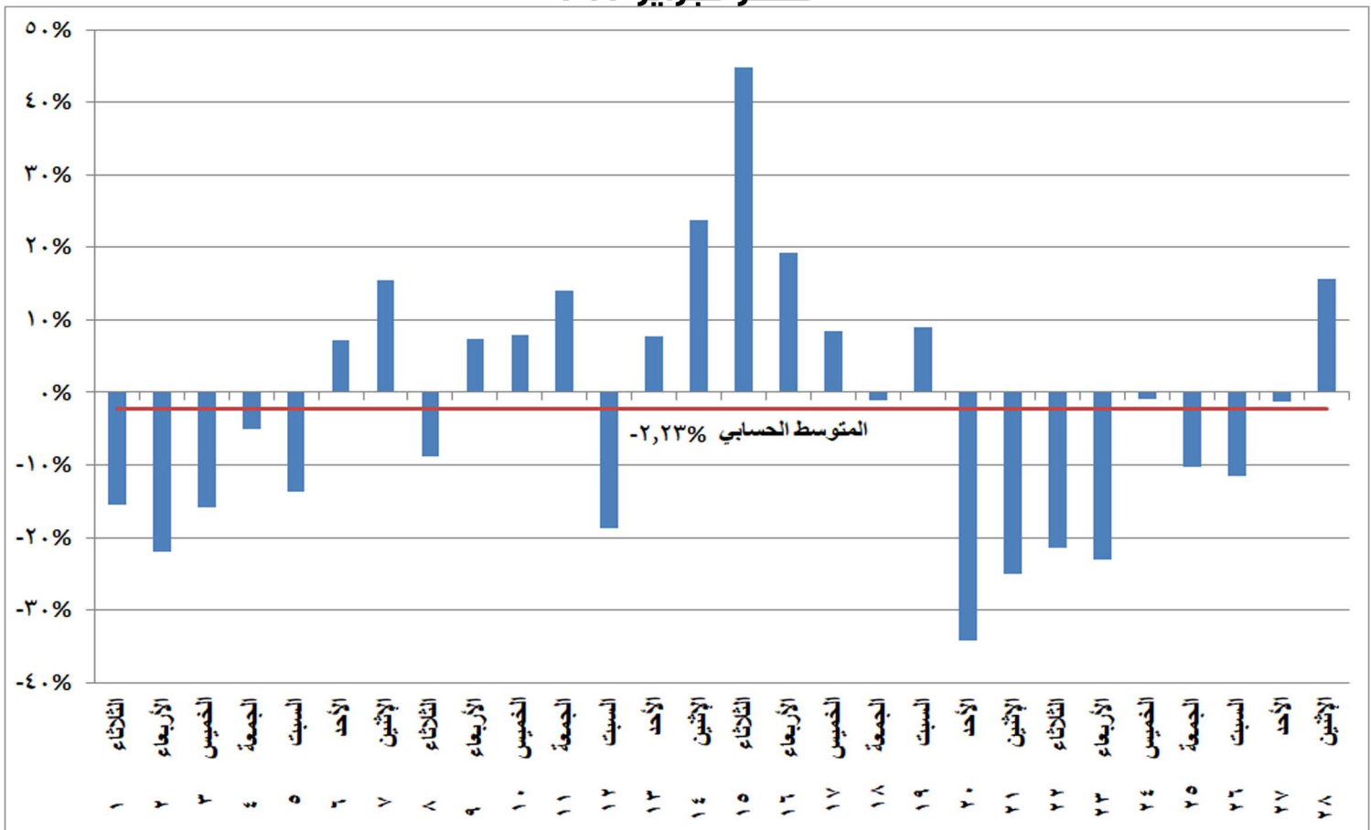
شكل (٢٢) نسب التغير في استخدام المصادر غير الحرارية في إنتاج الطاقة الكهربائية خلال شهر فبراير ٢٠٢٢ مقارنة بالشهر المماثل من العام السابق
